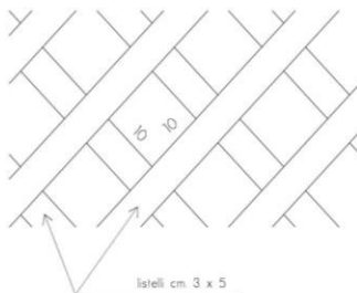
PARTICOLARE GRATICCIO
