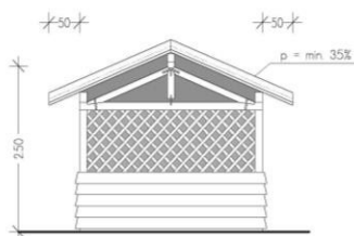
PROSPETTO LATERALE
