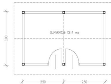
PIANTA
