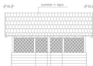
PROSPETTO
