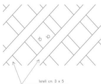
PARTICOLARE GRATICCIO
