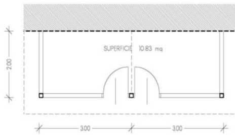
PIANTA
