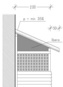
PROSPETTO LATERALE
