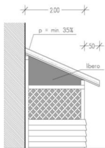
PROSPETTO LATERALE
