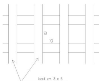
PARTICOLARE GRATICCIO
