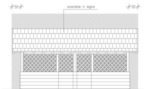
PROSPETTO
