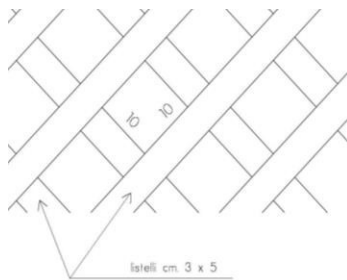
PARTICOLARE GRATICCIO
