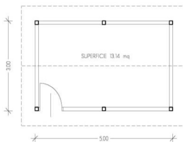
PIANTA
